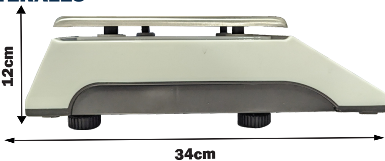
VISTAS LATERALES
